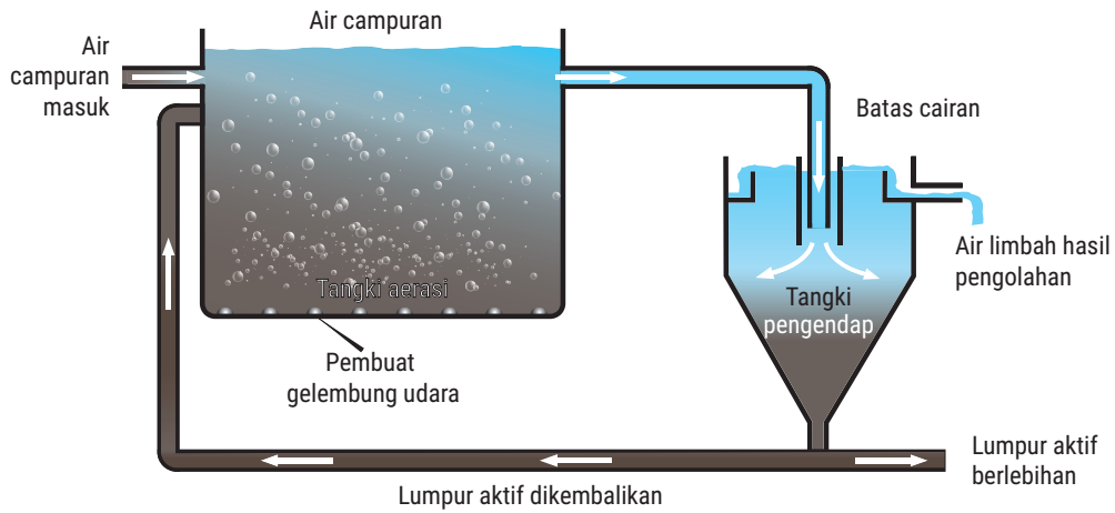
Gambar 4.1 Teknik bioremediasi pada IPAL.
